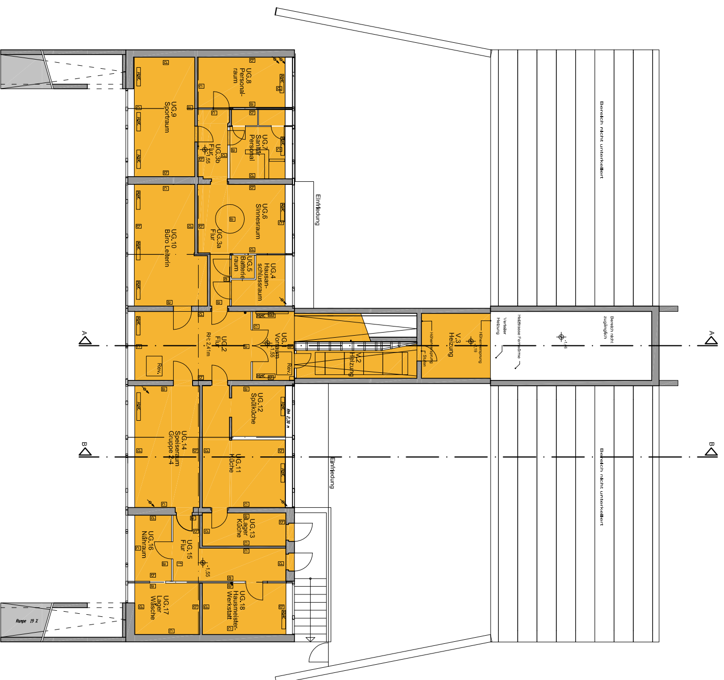
Ostflügel - Untergeschoss
